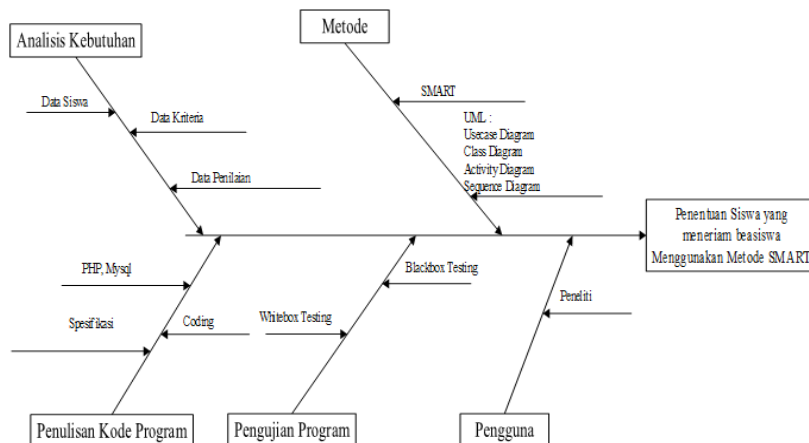
Gambar 1. Kerangka Fishbone
